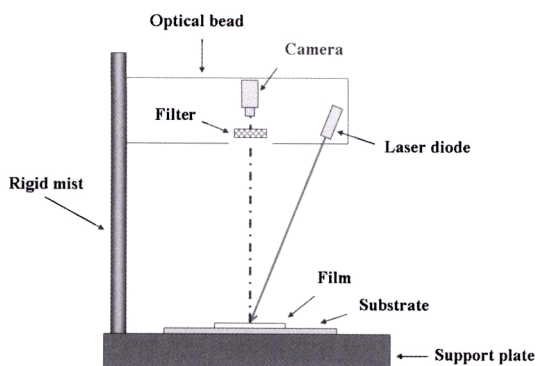
Fig. 1. HORUS film formation analyser.
